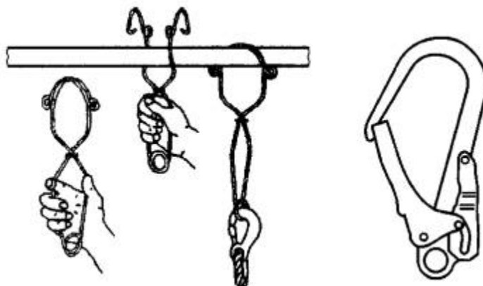
Рисунок 3 - Пример анкерных соединительных элементов (класс А)
