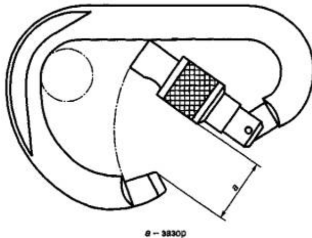
Рисунок 5 - Пример зазора в запорном элементе
